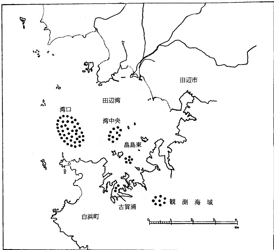
図1 調査海域
