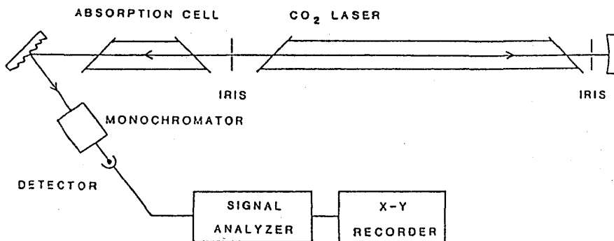
図1 装置図
