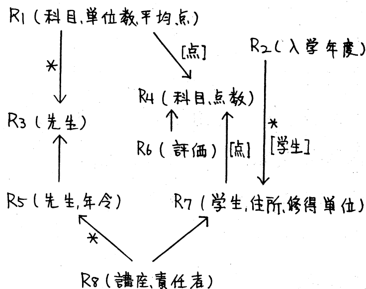
図7 データベースの設計(II)
