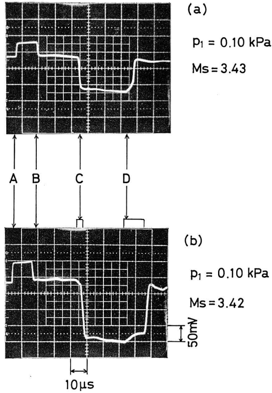
Fig. 9. Output Signal.
