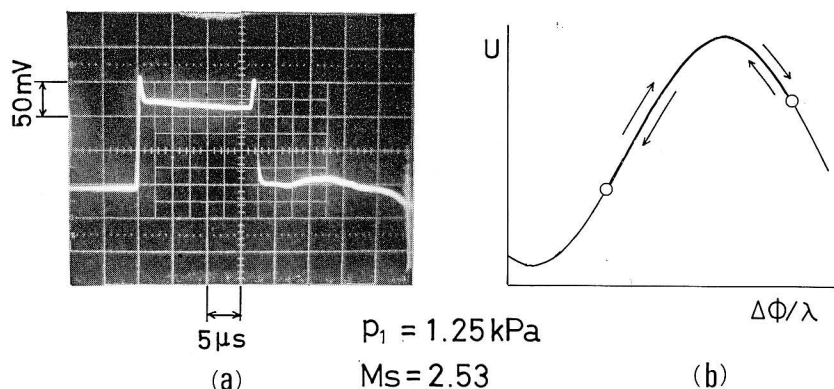
Fig. 7. Output Signal.
