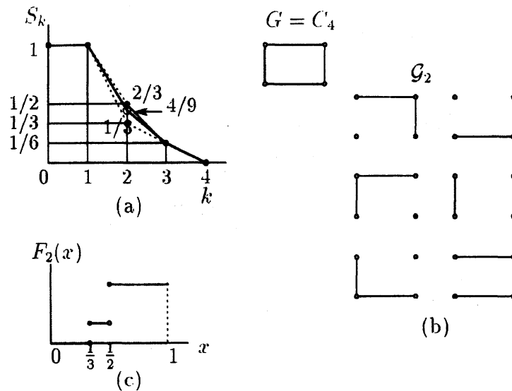
図 1: サイクルグラフ C_4 の例. (a) 横軸は除去する枝の数 k をとり, 縦軸に S_k のとり得る値を示す. 実線の折れ線は期待安定連結関数の値を結んで示したもの. k=2 のとき S_k は 2 種類の値をとる. (b) k=2 のときの \mathcal{G}_k の全要素. (c) k=2 のときの S_k の累積分布関数.
