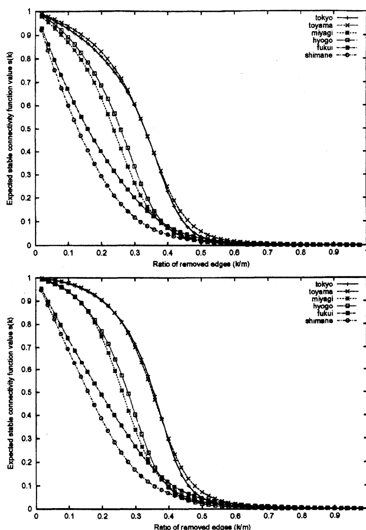
図 3: 6 都県（東京都，富山県，宮城県，兵庫県，福井県，島根県）の道路網の期待連結安定関数（上），次数 1 の頂点を除いたグラフの期待連結安定関数（下）
