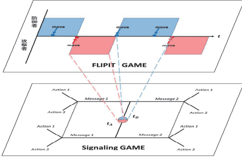
図 1: CCG モデル
