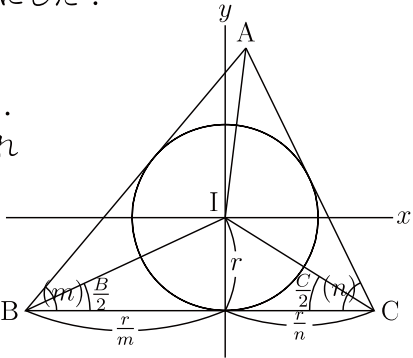
図 2. mnrf 法
