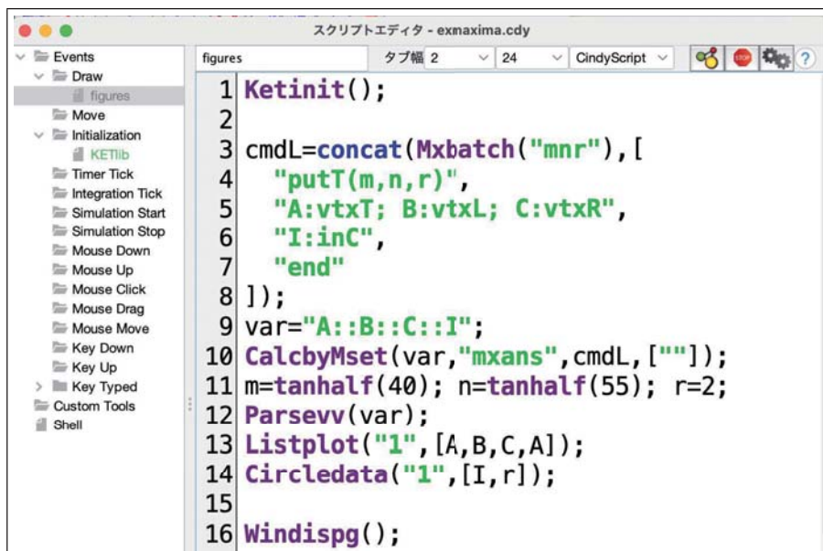
図 3. CindyScript の画面
