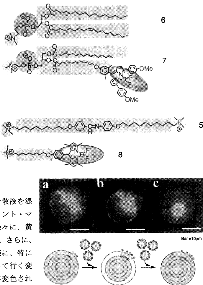
図5 ジャイアントベシクル膜の蛍光変色
