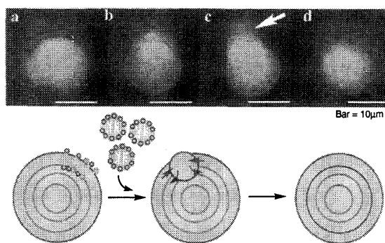
図6 双頭極性型両親媒性分子の膜内相分離現象
