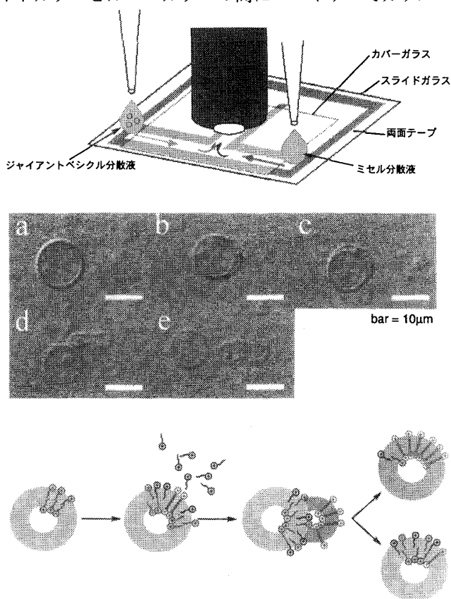
図 4 カナル型混合プレパラートと脱水縮合反応によるジャイアント母ベシクルの分裂のリアルタイム観察像及びその模式図
