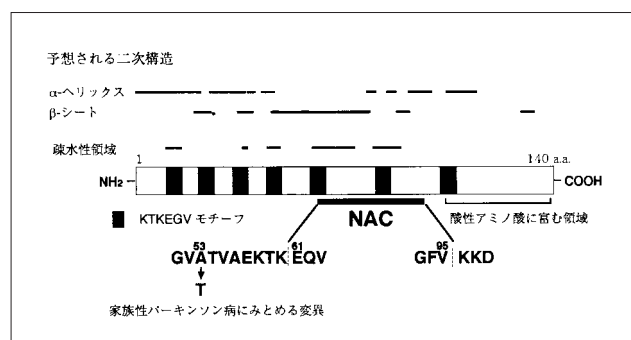
図. NACP/ \alpha -シヌクレインの構造と変異部位
