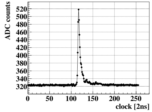
(b) 500-MHz sampling ADC
