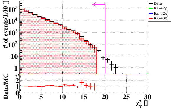
(e) \chi^2_z
