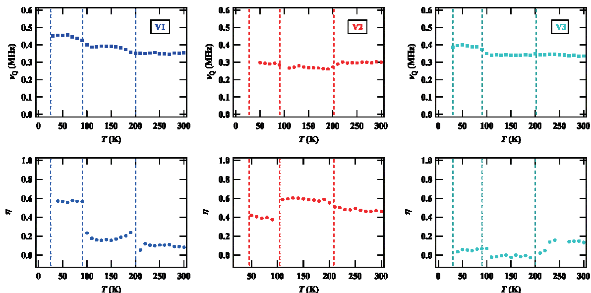
図5 各バナジウムサイトの核四重極周波数 \nu_Q と異方性パラメータ \eta の温度依存性。
