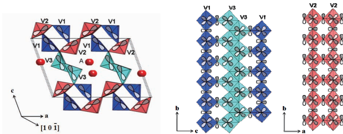
図 2 \beta - \text{Ag}_{0.33}\text{V}_2\text{O}_5 のラダー構造。
