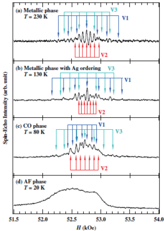
図3 H \parallel b , 59.00 MHz における磁場掃引 ^{51}\text{V} NMR スペクトル.
