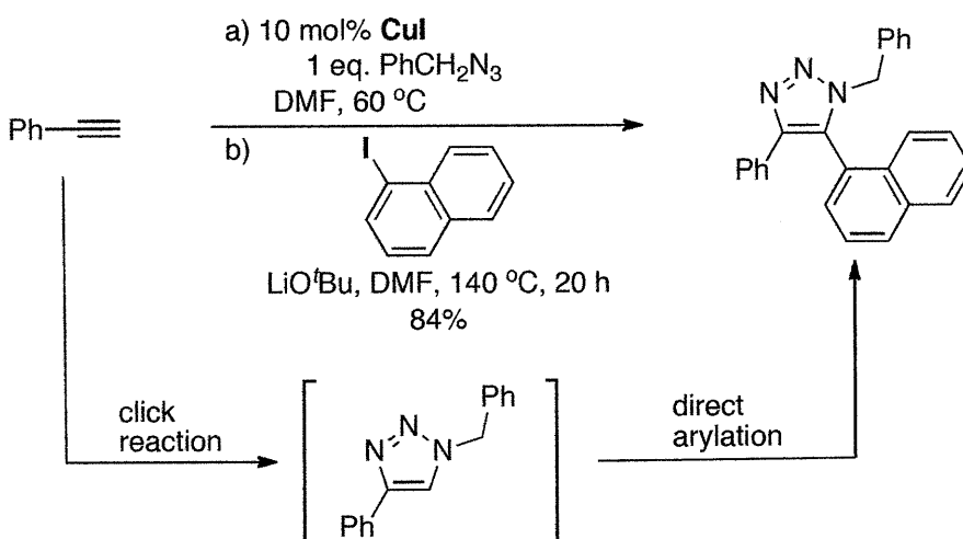
Scheme 23.
