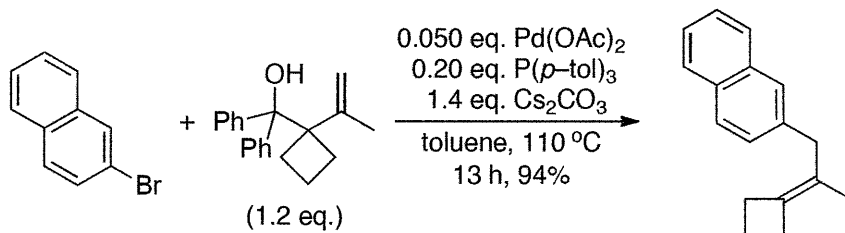
Scheme 31.
