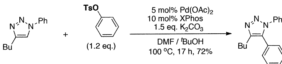
Scheme 22.
