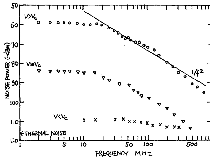
図2. 雑音スペクトル 1)
