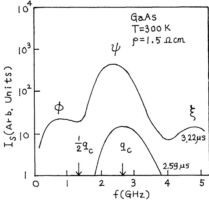
図4. 増幅フォノンのスペクトルの時間発展 14)
