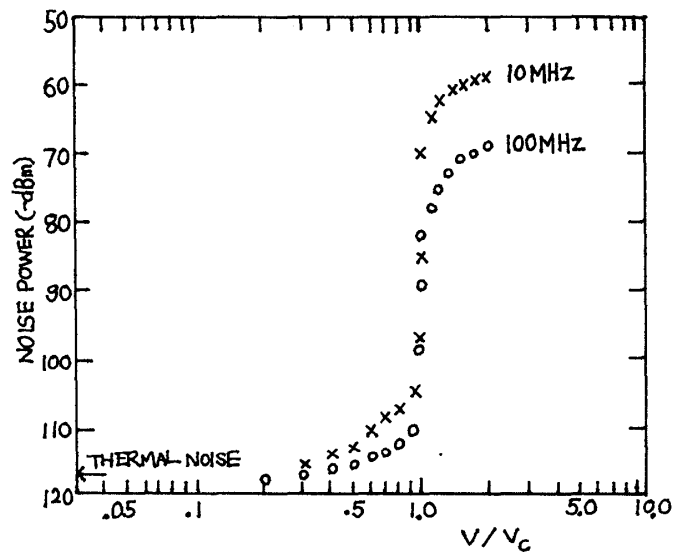
図1. CdS の電流雑音 1)
