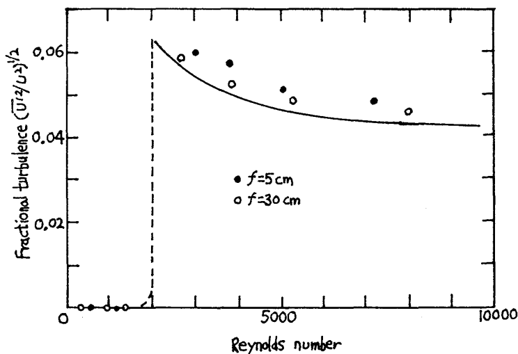
図 3. 乱流の揺らぎ 8)
