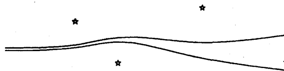
図 1: 2 つのテスト粒子の軌道
