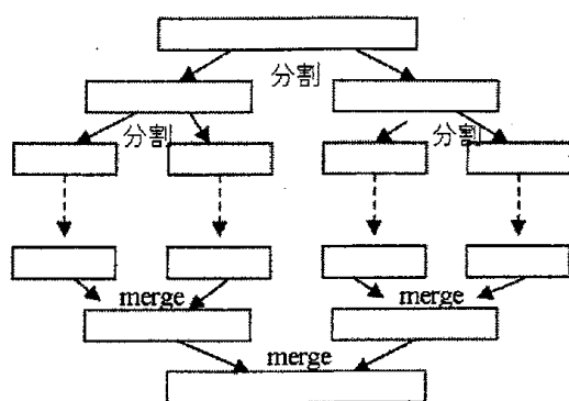
図 4: マージソート
