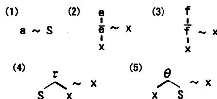
図 1: 還元規則
