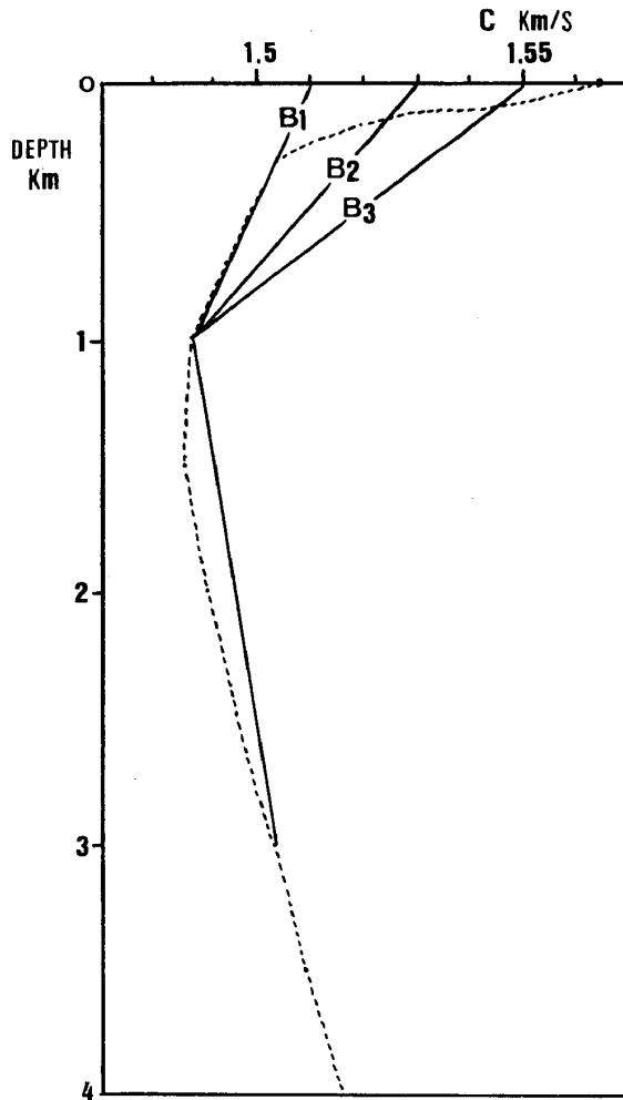
図8 海中音速鉛直分布のモデルB (a) モデルB 1 (b) モデルB 2 (c) モデルB 3
