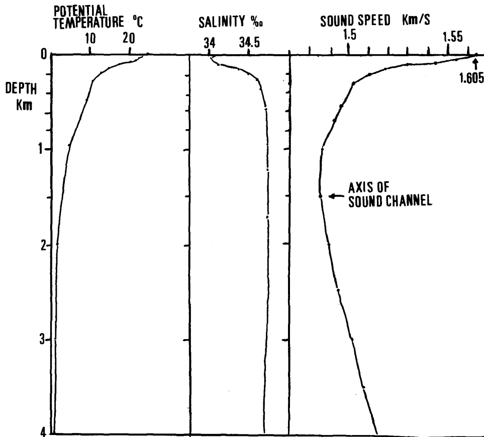
図5 インド洋の10°S, 110°Eにおけるポテンシャル水温・塩分の分布 [National Science Foundation 1971] とそれにもとづいて計算された海中音速鉛直分布
