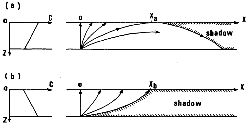
図1 海中音速の伝わり方
