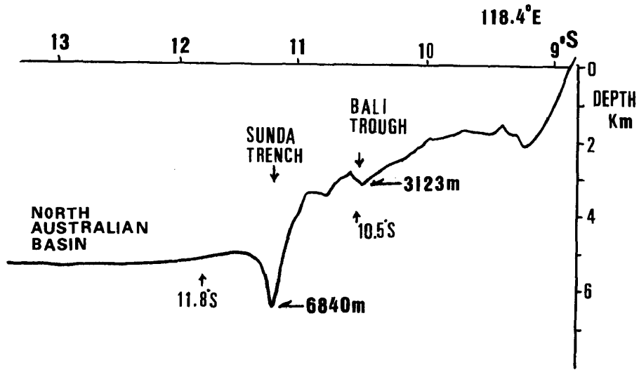
図4 観測測線118.4°E沿いの深浅測量断面図 ただし、測線の位置は図3に破線で示した。
