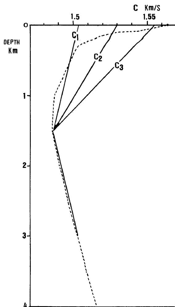
図10 海中音速鉛直分布のモデルC
