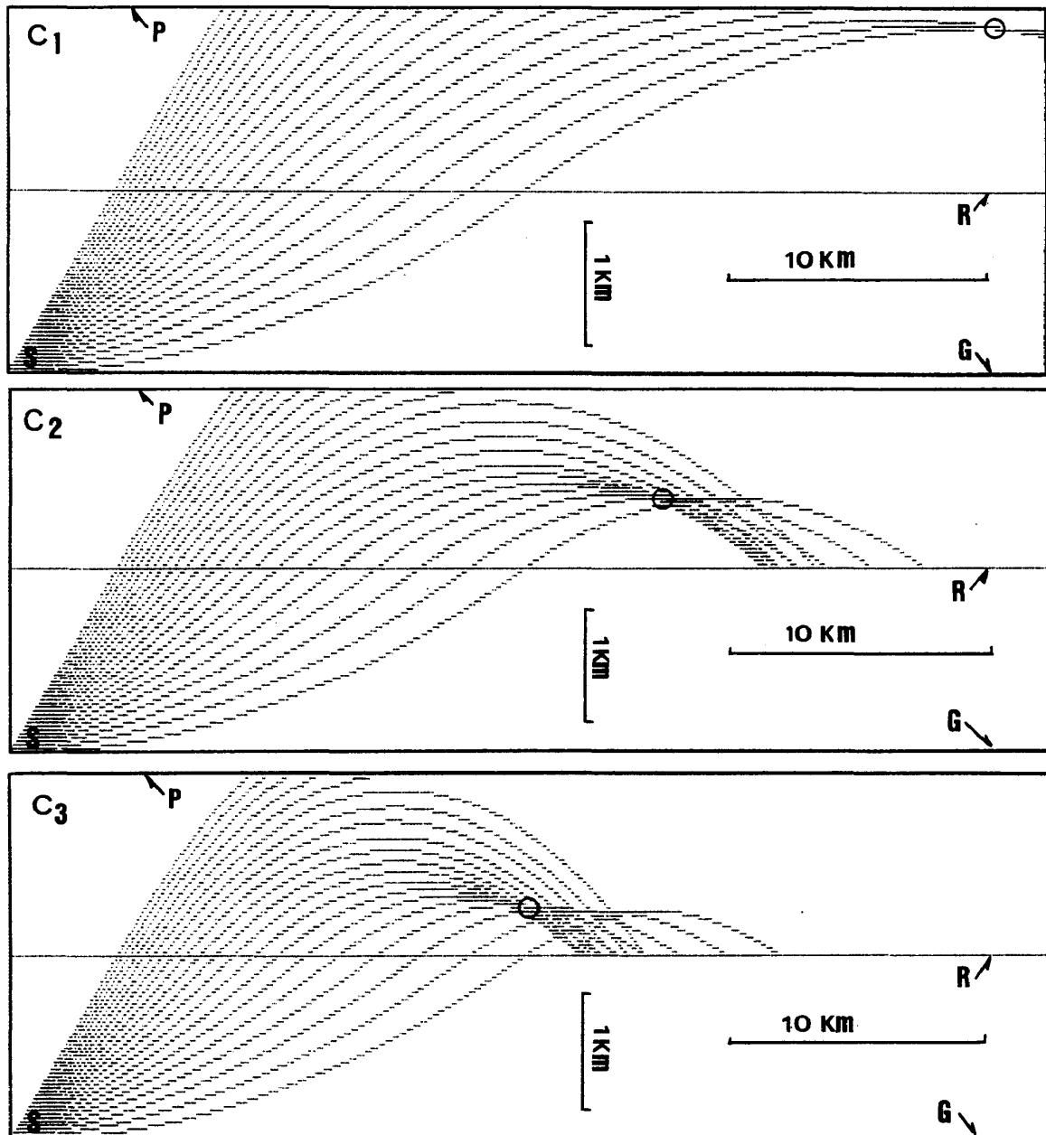
図11 モデルC に対する海中音波の径路の計算結果 記号説明などは図7に同じ。
