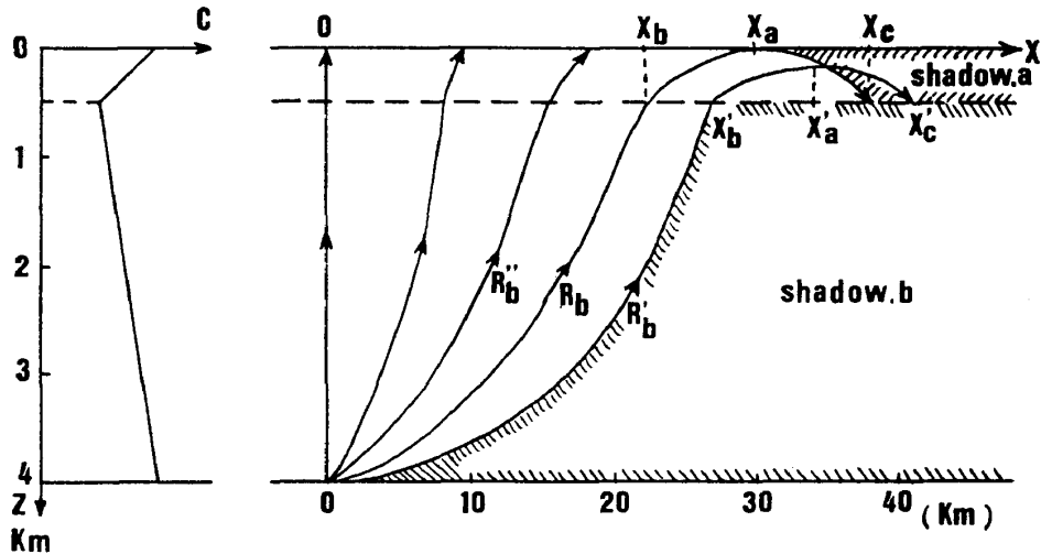
図2 ある海洋で海中音速の鉛直分布とそれに対する海中音波の伝わり方
