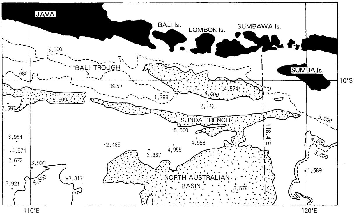
図3 スンバワ島南沖の海底地形
