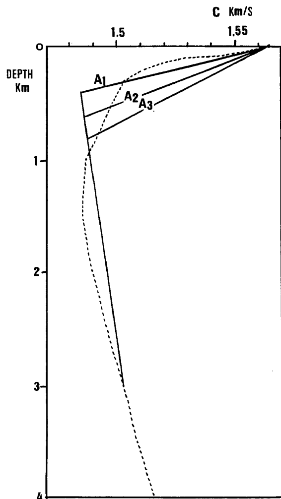
図6 海中音速鉛直分布のモデル A
