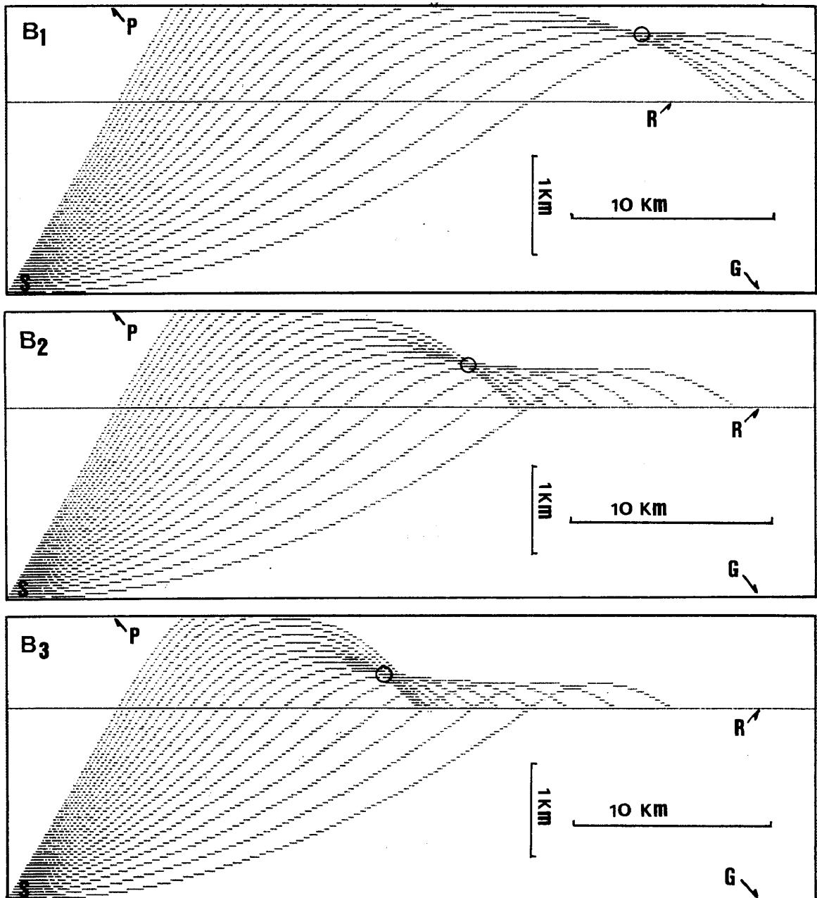
図9 モデルBに対する海中音波の径路の計算結果 記号説明などは図7に同じ。
