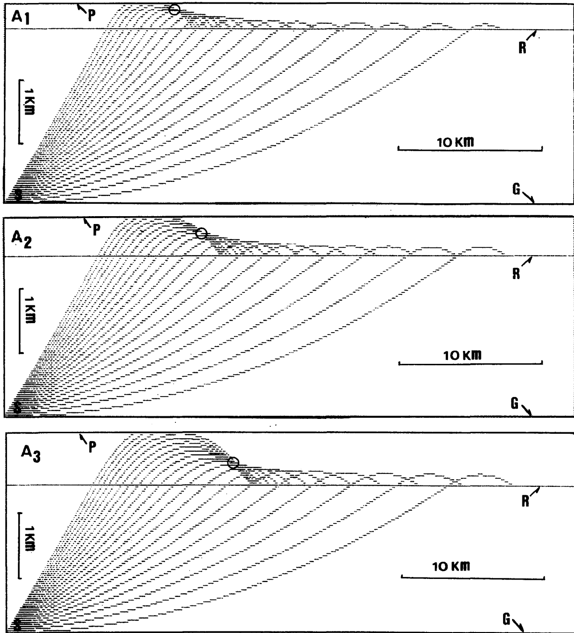
図7 モデルAに対する海中音波の径路の計算結果
