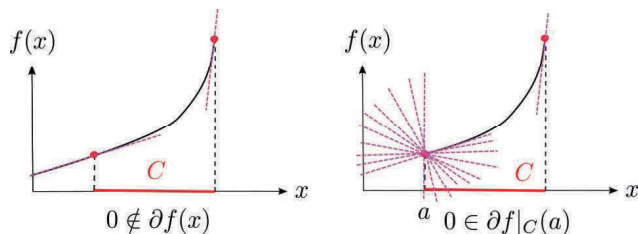
図 1: \partial f(x) \subset \partial f|_C(x) .
