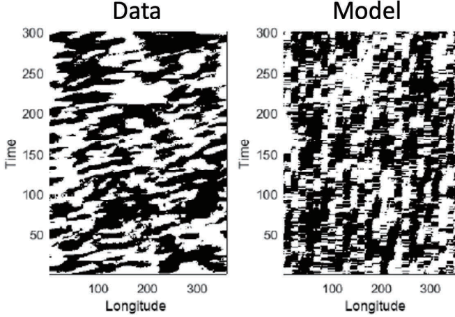
図 4: 観測データ (左) とモデル (右) の時空ダイアグラム.
