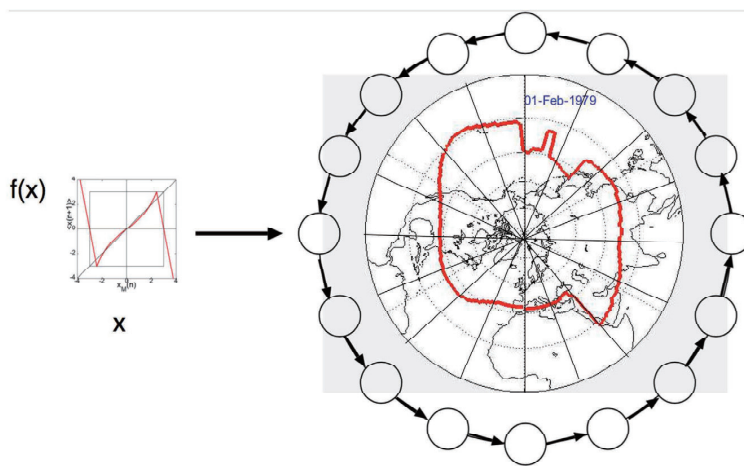
図 3: 中緯度ジェット気流のミニマルモデル
