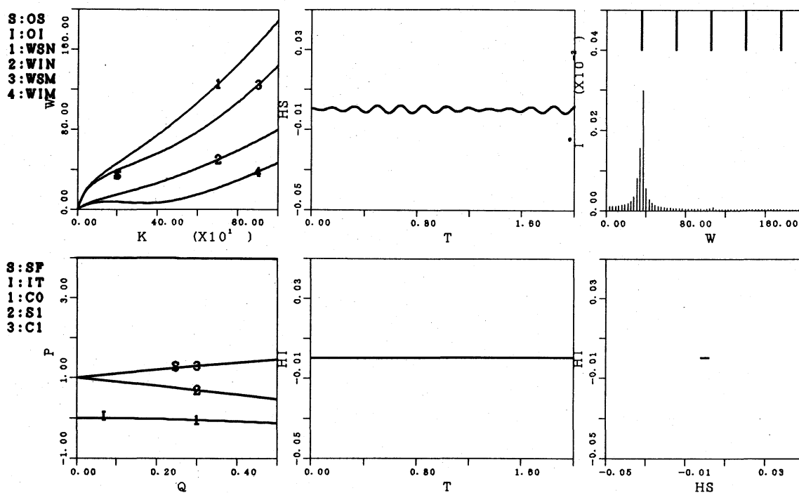
図 3: Normal Mode 方程式の数値解: \Omega = 35.0 \text{ s}^{-1}
