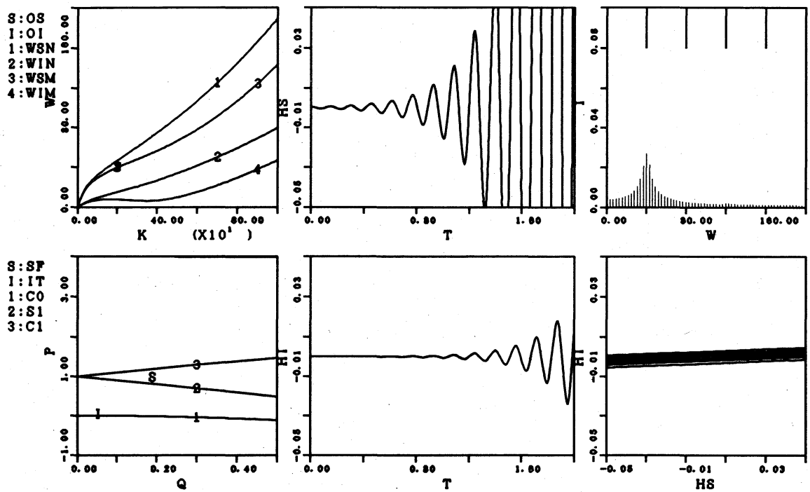
図 4: Normal Mode 方程式の数値解: \Omega = 40.0 \text{ s}^{-1}
