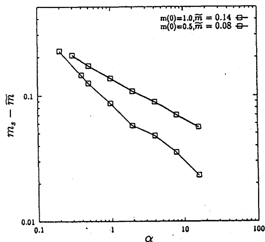
図 5: N \rightarrow \infty での m_s の \alpha 依存性 ( m(0) = 0.5, 1.0 )。 \bar{m} = 0.14 は Kinzel の結果と一致する。
