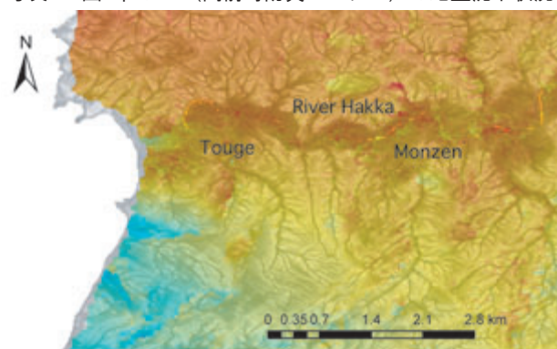
図3：門前～道下地区のハケ川沿いとその周辺地域の D_{insar} 分布図と TWI 分布図。濃い灰色の地盤湿潤度の高い部分は D_{insar} 大の濃い赤部分と良く一致。
