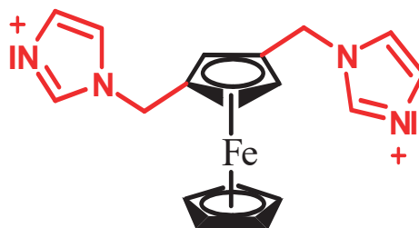
新規 IL (a) の化学構造
