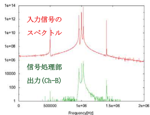
図2：Ch-B出力
