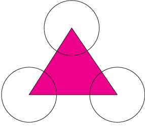
図 1: 円板 3 枚の非交和の minimal unfolded region
