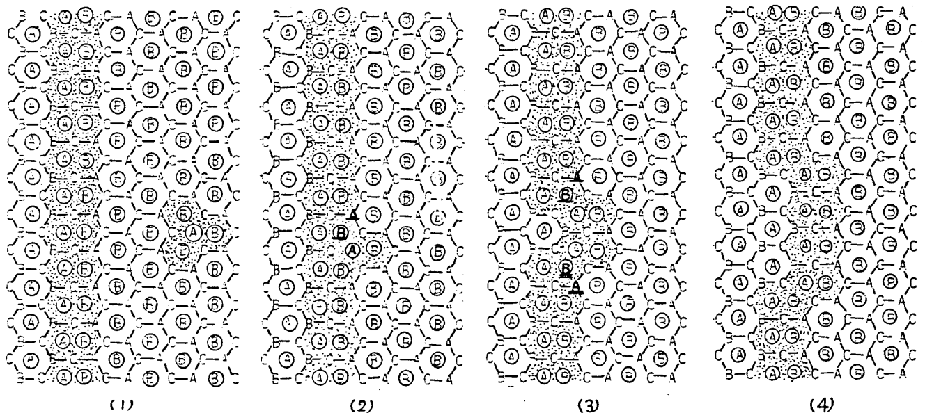
図5 梯子状境界と一個の自由な乱れの振舞の例
