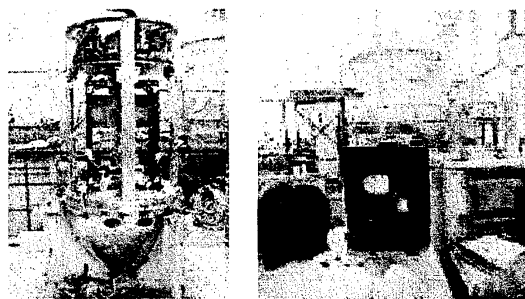
図 13 実験装置を組み込んだ落下カプセル（左）と、真空中の落下をモニターする様子
