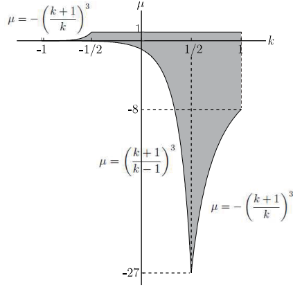
Figure 3: \omega = 3 の場合の安定領域。
