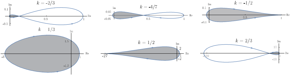
図 1: 複素平面における B_{3,k}(\theta) のグラフと領域 D_{3,k}^\gamma(0) .
