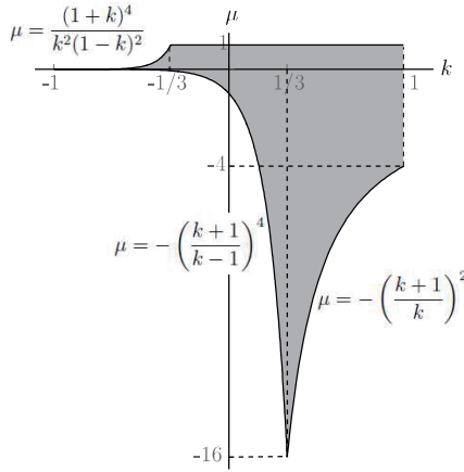
Figure 2: \omega = 4 の場合の安定領域。
