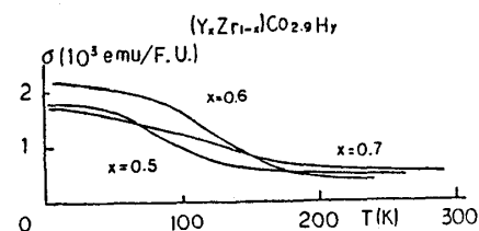
図3 (Y x Zr 1-x )Co 2.9 ( 0.7 \geq x \geq 0.5 ) 水素化物の磁化
