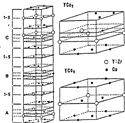
図1 PuNi 3 構造とcubic Laves R 2 T 4 およびCaCu 5 RT 5 格子
