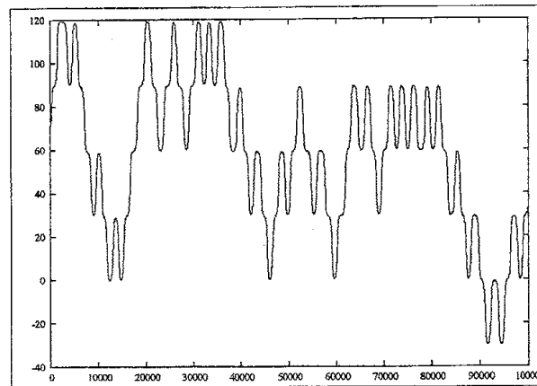
図 6: 乱歩パルスの位置の時間変化. 空間的な非一様性は周期的であるが, パルスの運動はその進行方向をランダムにかえるものとなる場合がある. 数値的に得られたパルスの運動の統計的な解析により, この運動はブラウン運動と同値である事がわかっている. ( F = 0.018, k = 0.052, \epsilon = 1.02, d = 2, L = 500, l = 30, b = 0.18 )
