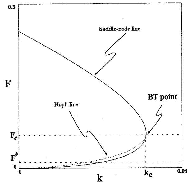
図 2: サドル・ノード分岐を実線であらわし, ホップ分岐を点線であらわす. これら 2 線は余次元 2 の分岐点である Bogdanov-Takens 点で交わる.
