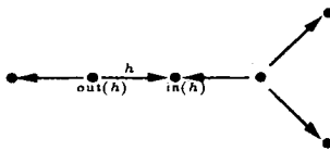
図 1. quiver の例
