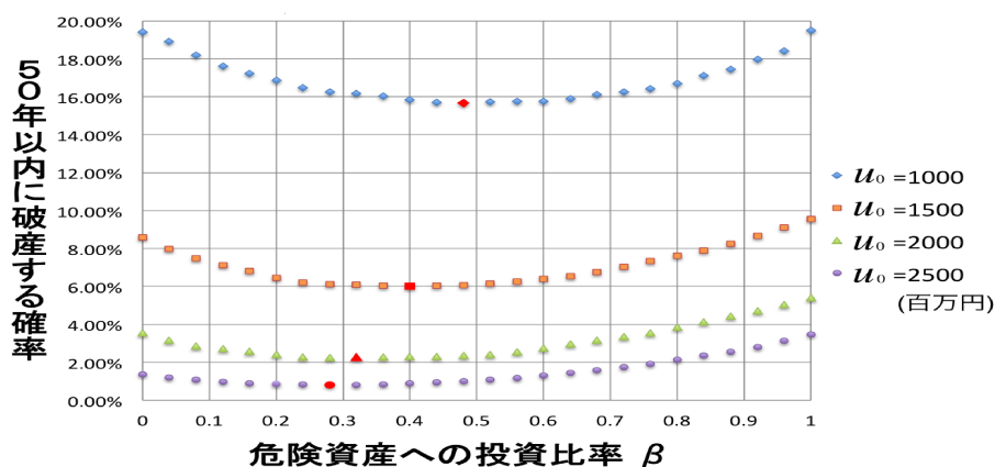
図 2: 初期サープラス u_0 だけを変化させた場合の影響
