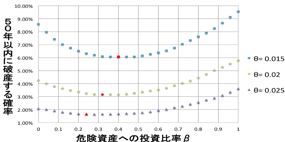
図 3: 安全割増率 \theta だけを変化させた場合の影響
