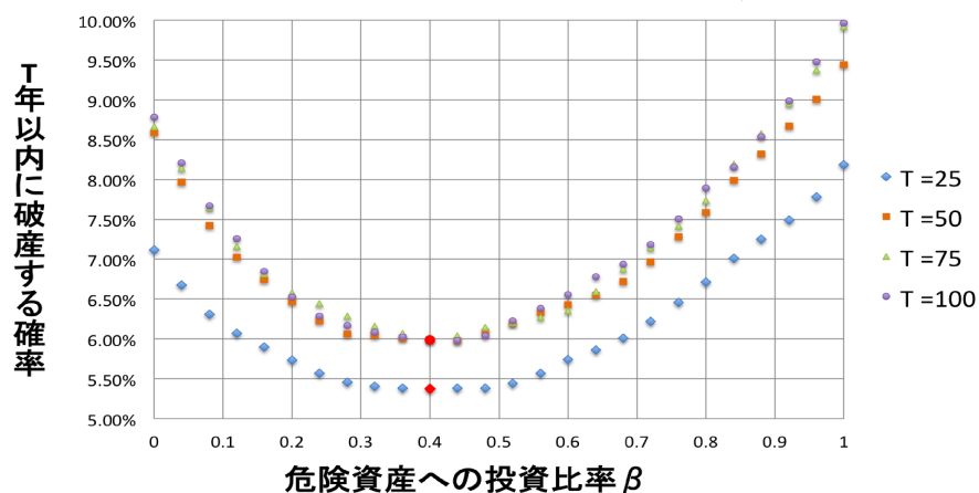
図 4: シミュレーション期間 T だけを変化させた場合の影響
