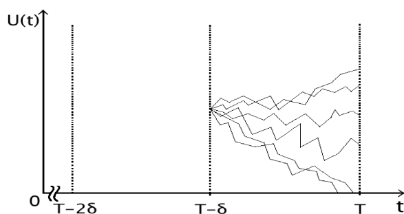
図 6: 破産確率算出のイメージ図
