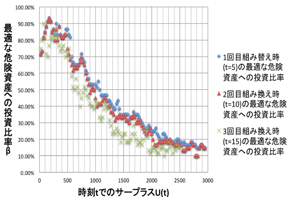
図 7: シミュレーション結果
