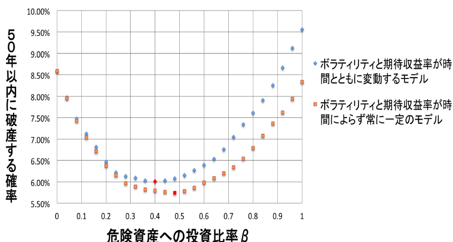
図 5: モデル比較のシミュレーション結果
