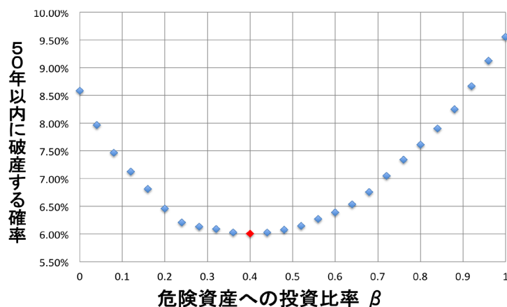
図 1: 破産確率のシミュレーション結果
