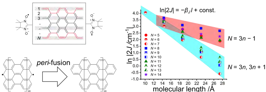
図1. (a) AGNRs の幅 N の定義と両端に置換するニトロニルニトロキシド (NN) (b) エッジ由来のスピンを打ち消すペリ縮環 ( N = 7 の系を例示) (c) NN 間交換相互作用 J の分子長依存性
