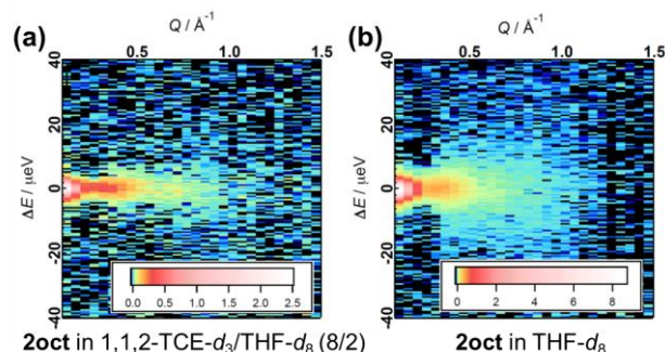
図2. (R)-2-オクチルオキシメチル基を有する PQX (2oct) の中性子準弾性散乱測定結果。(a) 重水素化 1,1,2-TCE/重水素化 THF 混合溶媒 (4/1, v/v), (b) 重水素化 THF 溶液。
