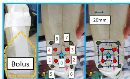
図 1. 照射試験時の足部ファントム
