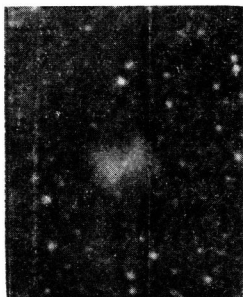
M27 小狐座14の南半度にある亜鈴状星雲。露出20分。
