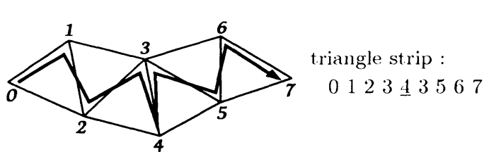
図 5: トライアングルストリップの縮退 : 1 縮退の曲がるパターン
