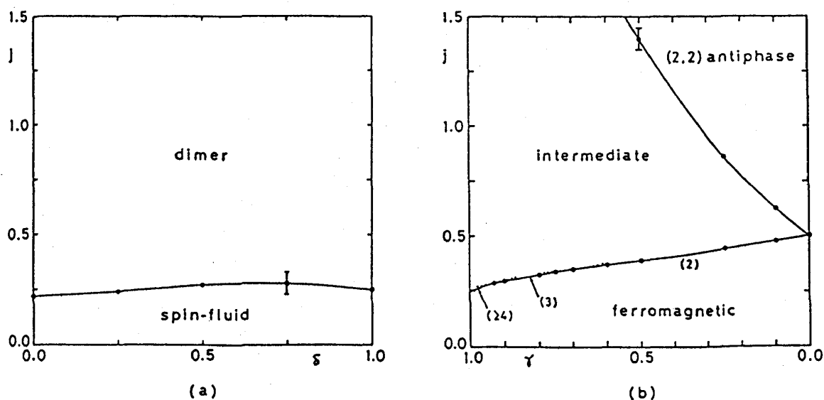
図 2 J_1 < 0 のときの無限系の基底状態の相図. (a) 相互作用の異方性が XY 型の場合 ( \gamma = 1 , 0 \leq \delta < 1 ), (b) 相互作用の異方性が Ising 型の場合 ( 0 \leq \gamma < 1 , \delta = 1 ).
