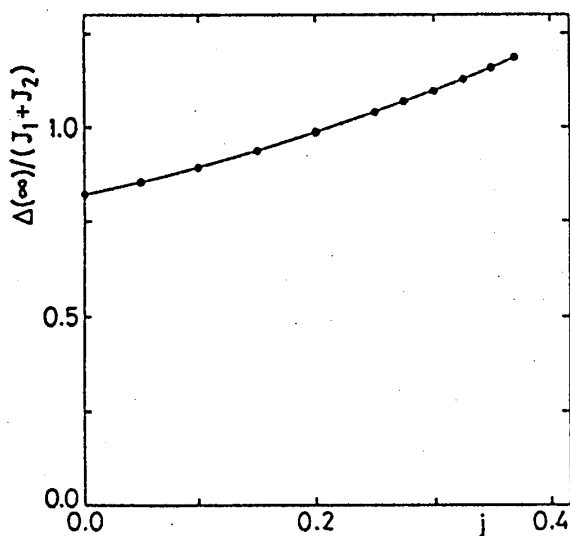
図 3 (左図) \Delta(\infty)/(J_1+J_2) の j 依存性.
