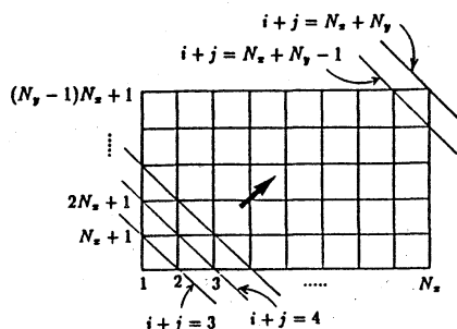
図1 2次元超平面法
