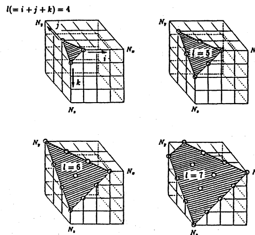
図2 3次元超平面法における超平面
