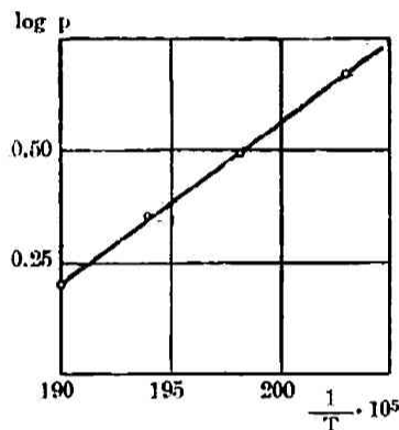
限界壓と溫度との關係 第十二圖
