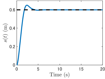
(d) the position of the slider s(t)
