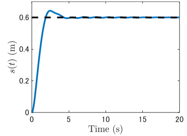
(d) the position of the slider s(t)
