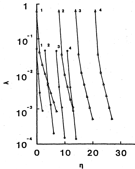
図3 Grad-Shafranov方程式を解いた時の収束の速さ 縦軸: \lambda は残差を、横軸: \eta は緩和の回数を示す。 「 \Delta 」印は Fourier 変換後、緩和法だけで解いた場合。 「 \circ 」印は長波長成分を直接法で解き、残りを緩和法で計算した場合。どちらの場合も、過緩和法は用いないが、 \alpha (加速係数=0)。また書き込まれている小さな数字は Newton 法の回数である。
