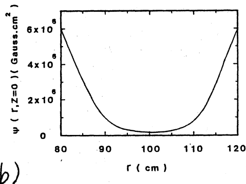
図4 Grad-Shafranov 方程式の数値解析結果
