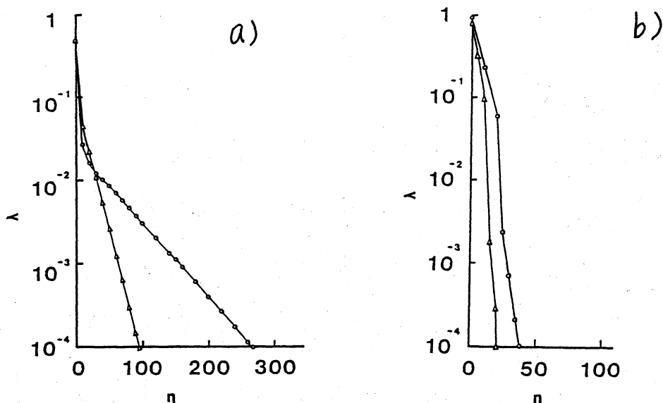
図1. 微分方程式(18)を解いた時の収束の速さ
