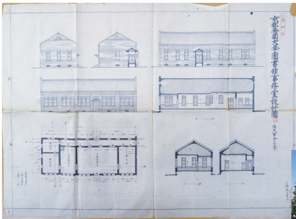
京都帝国大学図書館事務室設計図 (京都大学施設部所蔵)
