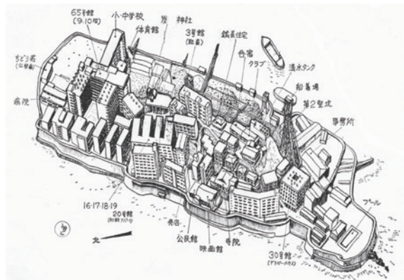
軍艦島島瞰図（西山のスケッチ） 西山は1952年と1970年に長崎県の端島炭鉱の住み方調査を実施した。稼働中の島内を踏査し、カメラに収めた。
