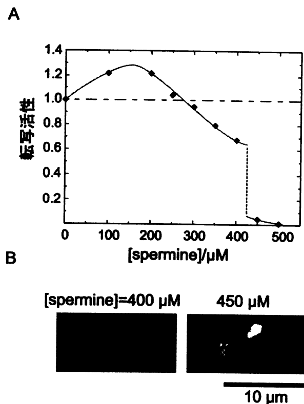
図 1. 転写活性のスイッチング。(A)スぺルミン濃度に依存した転写量の変化. ZAPII DNA (40 kbp, T7 プロモータをもつ)を T7 RNA ポリメラーゼにより、37℃で 1 時間転写した後、転写産物を蛍光強度 (RiboGreen) で定量。[spermine] = 0 μM における転写産物量を基準とする。(B)λ ZAPII DNA の蛍光顕微鏡像。溶液と平衡にあるガラス表面上の DNA を DAPI で可視化。
