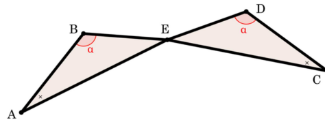
図 3.3. 性質 3.7 の図形
