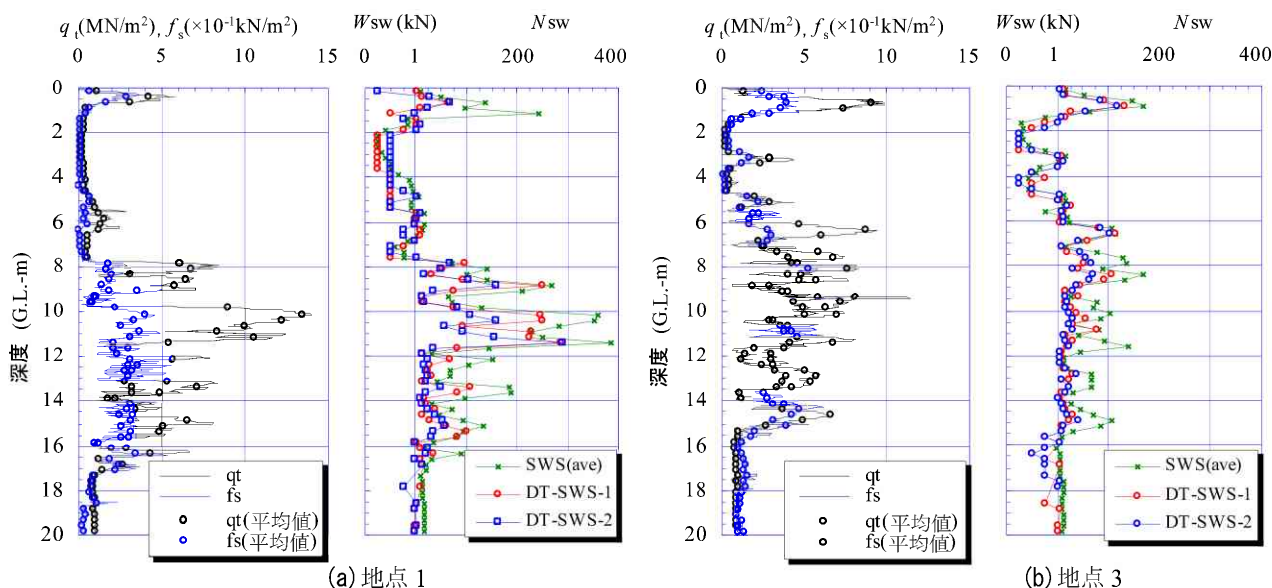
図7 q_t , f_s , W_{sw} および N_{sw} の深度分布
