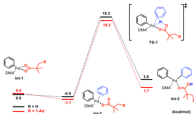
スキーム 2. C-H 結合切断過程の反応座標 (wB97XD/SDD for Pd, others for 6-31G(d))
