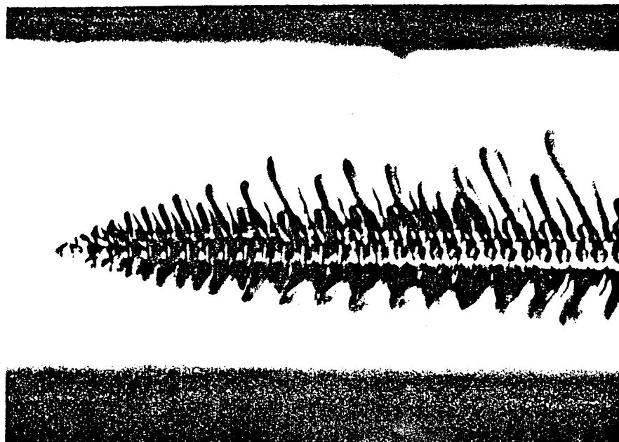
図1 (b) 毛細管中に成長する樹枝状結晶
