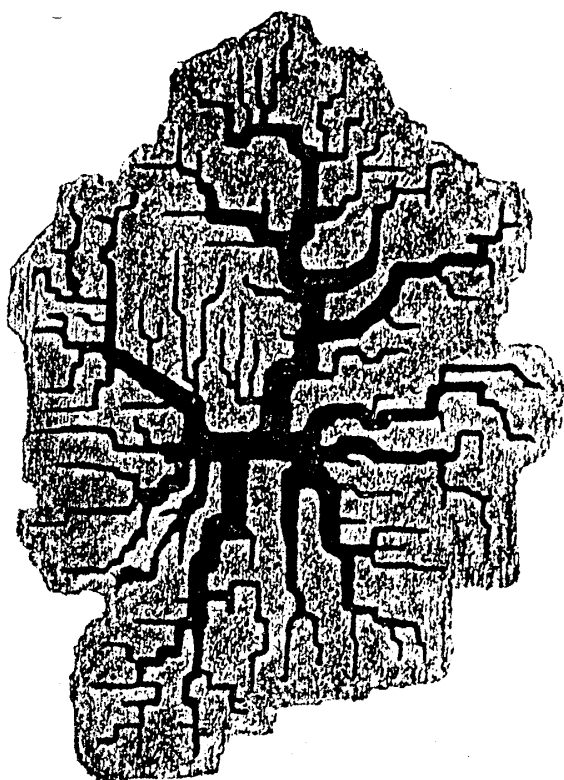
図2 (a) 絶縁破壊パターン計算機 シミュレーション r=1 ,
