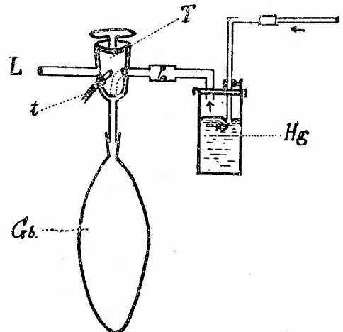
第三圖 過壓裝置裝用家兎ノ呼氣聚集裝置
