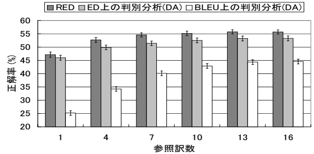
図 3 10 重交叉検定による性能比較。RED の性能 v.s. ED または BLEU による判別分析による自動評価の性能
