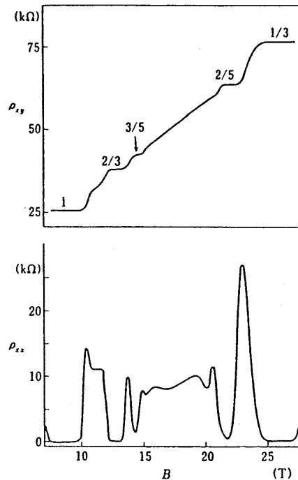
異常量子ホール効果の実験結果(Tsuiらによる) 結果は伝導度ではなく抵抗で与えられている。抵抗と伝導度の関係は、 \rho_{xx} = \sigma_{yy} / (\sigma_{xx}\sigma_{yy} - \sigma_{xy}\sigma_{yx}) , \rho_{xy} = -\sigma_{xy} / (\sigma_{xx}\sigma_{yy} - \sigma_{xy}\sigma_{yx}) となるので、 \sigma_{xx} = \sigma_{yy} (= \sigma_l) のとき \rho_{xx} = 0 , \rho_{xy} = 1/\sigma_{yx} = 1/\sigma_H
