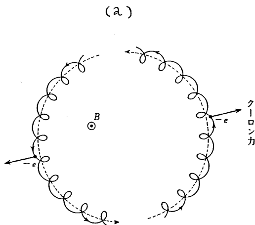
図 2 (b) 磁場中の2電子の運動(古典論)
