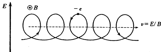
図 2 (a) 一様な電場、磁場中の荷電粒子の運動(古典論)
