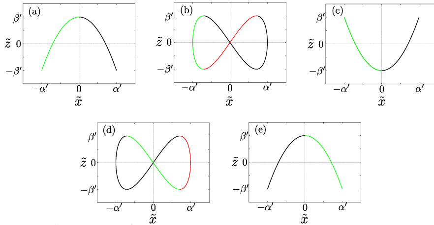
図 2: 容器の運動の軌跡図。(a) \gamma = 0^\circ , (b) \gamma = 45^\circ , (c) \gamma = 90^\circ , (d) \gamma = 135^\circ , (e) \gamma = 180^\circ . 赤色の線は 0 \leq t \leq \frac{\pi}{2\Omega} , 黒色の線は \frac{\pi}{2\Omega} \leq t \leq \frac{3\pi}{2\Omega} , 緑色の線は \frac{3\pi}{2\Omega} \leq t \leq \frac{2\pi}{\Omega} における軌跡を表す。
